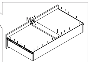
Fixação de fundo e reforço de gaveta
