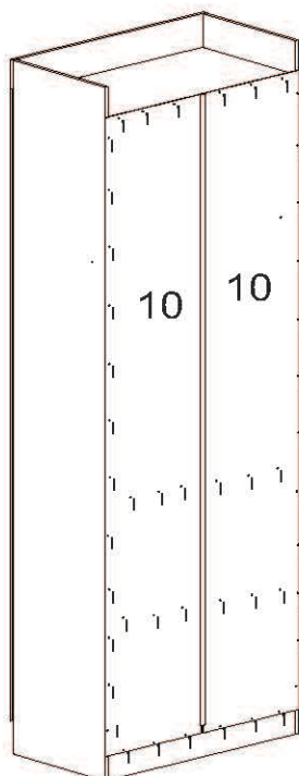
VISTA TRASEIRA
